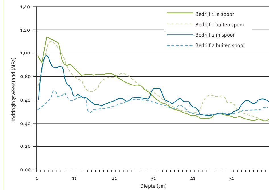
Figuur 2 Verskil indringingsweerstand in en buiten rijspoor van twee bedrijven.
